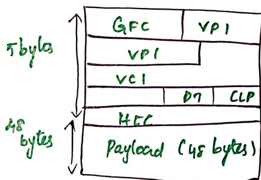
fig. UNI cell format
